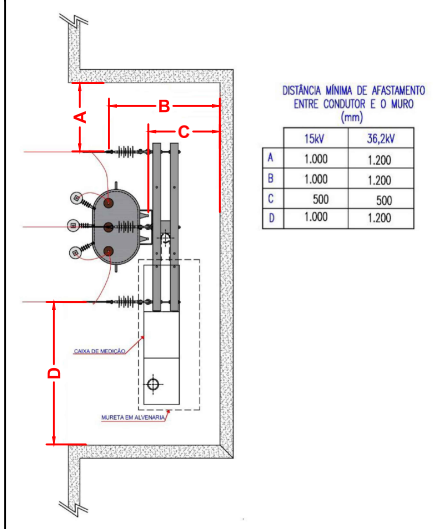
DETALHE DISTANCIAMENTO MÍNIMO NO RECUELO DA SUBESTAÇÃO
